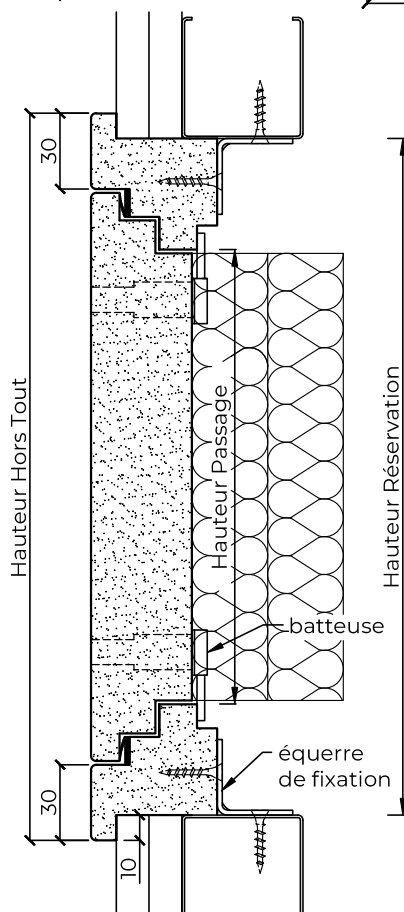
Coupe verticale
