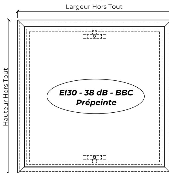
Élévation
