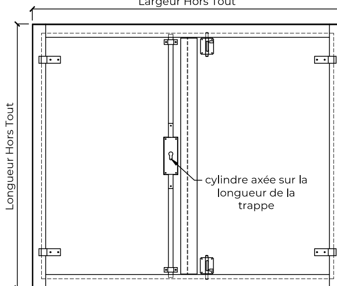
Elévation Largeur Hors Tout
