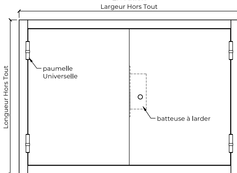
Elévation
