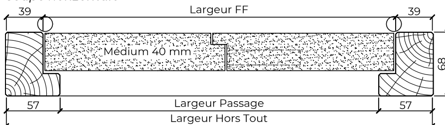
Coupe horizontale
