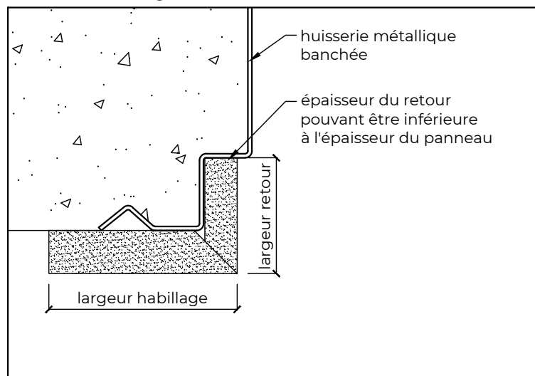
Profil de l'habillage sur huisserie banche
