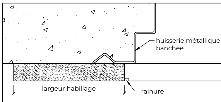
Profil de l'habillage sur huisserie banchée
