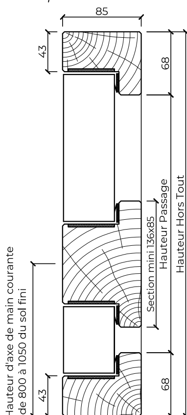
Coupe verticale
