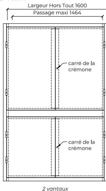
Elévation
