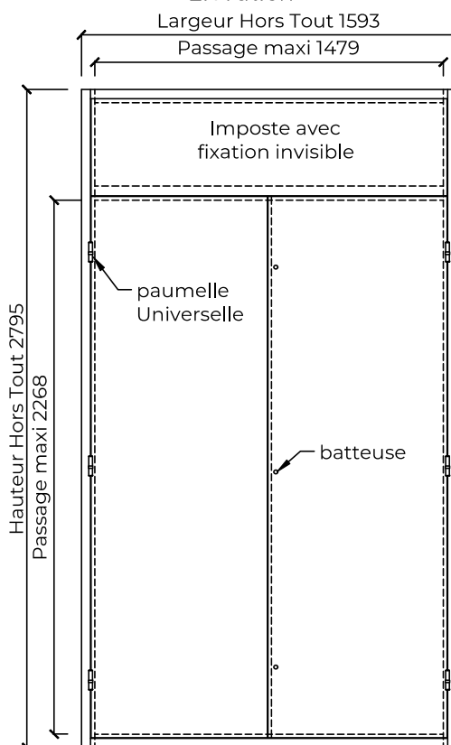
Elévation
