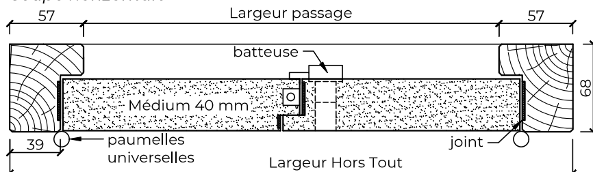
Coupe horizontale
