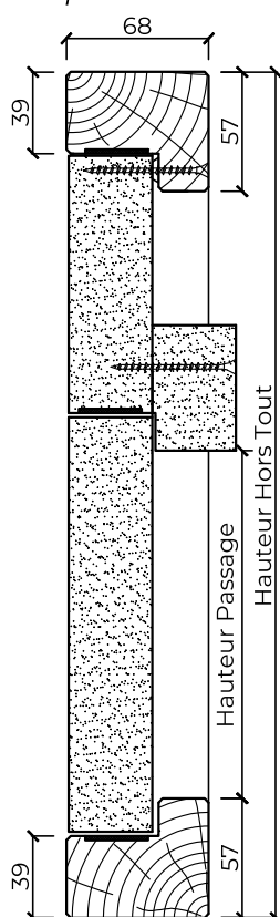
Coupe verticale
