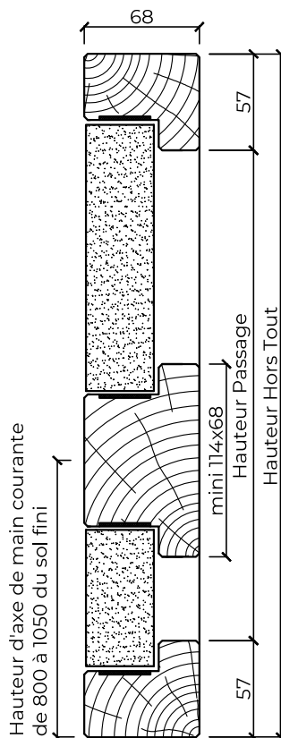
Coupe verticale
