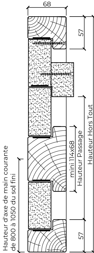
Coupe verticale
