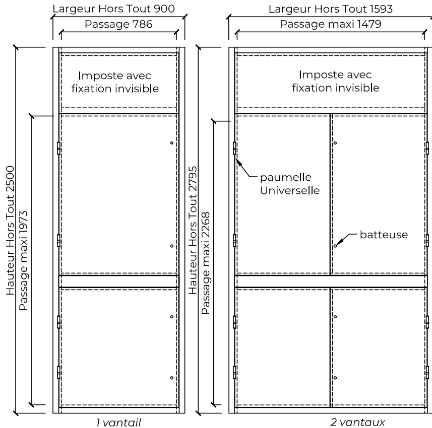
Elévation
