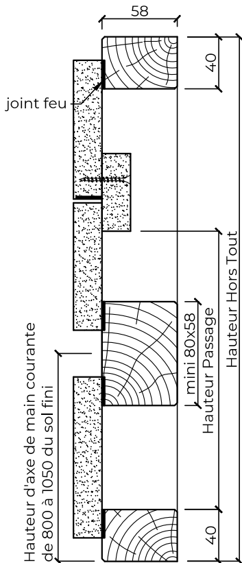
Coupe verticale
