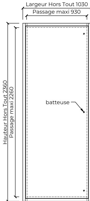
Elévation
