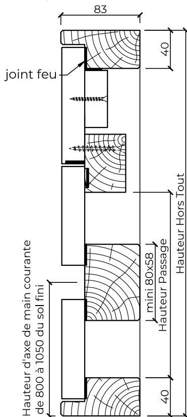
Coupe verticale
