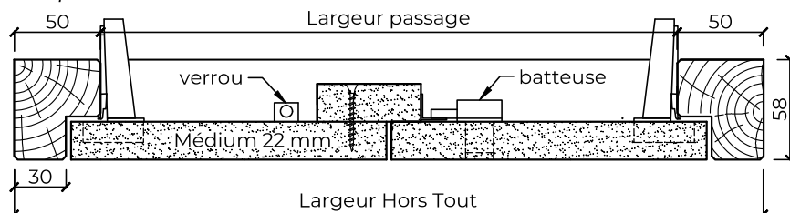
Coupe horizontale
