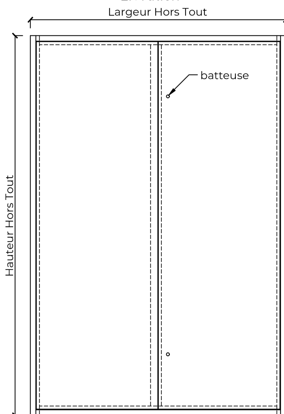
Elévation
