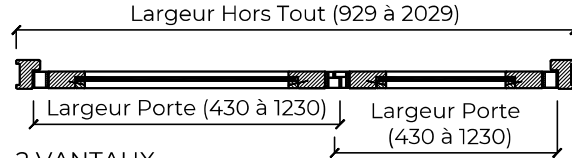
2 VANTAUX
