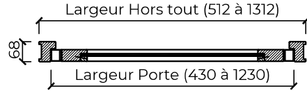
1 VANTAIL
