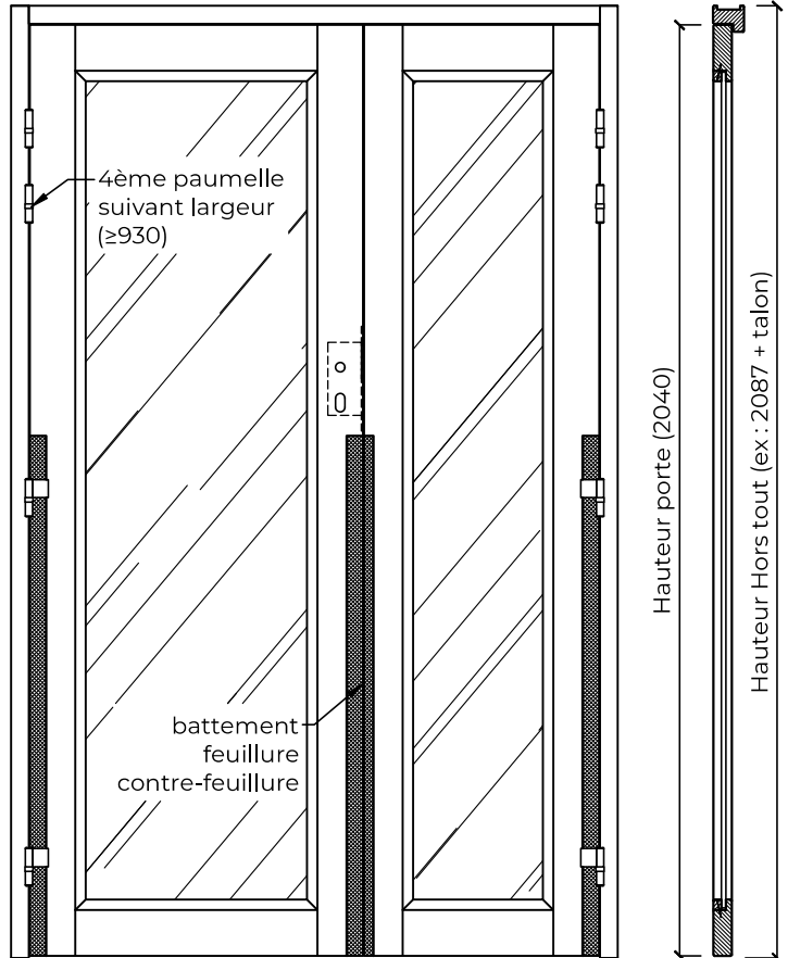
2 VANTAUX
