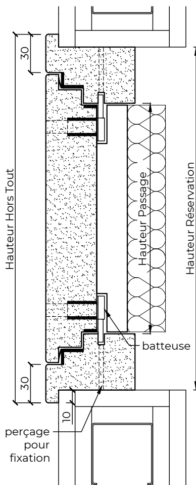
Coupe verticale
