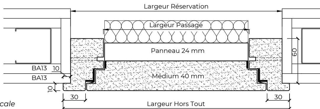
Coupe horizontale
