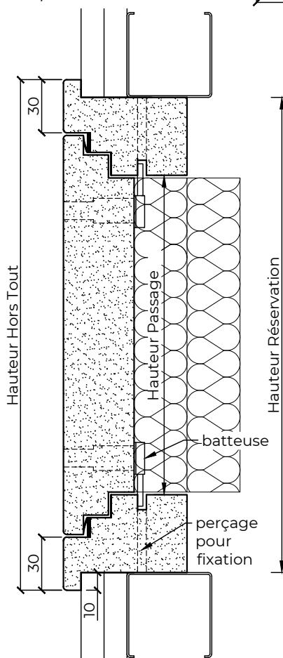
Coupe verticale
