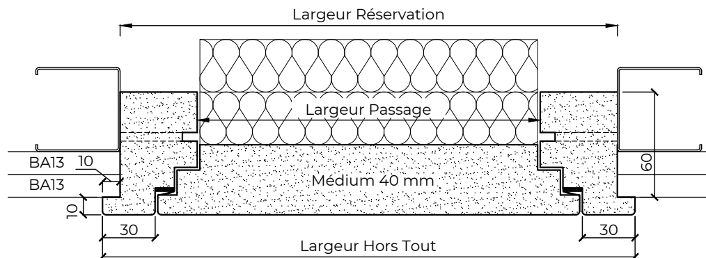
Coupe horizontale
