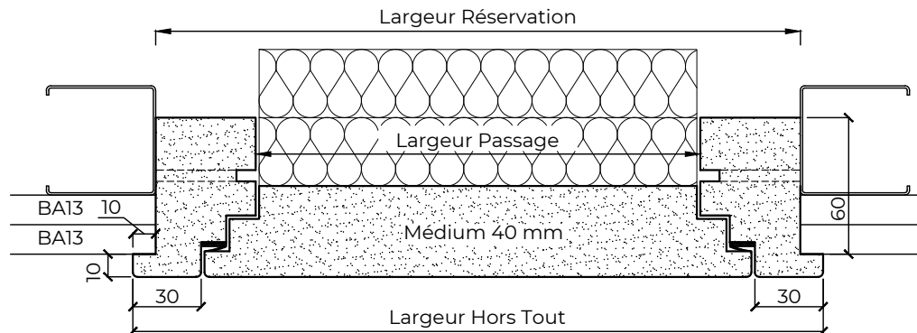
Coupe horizontale
