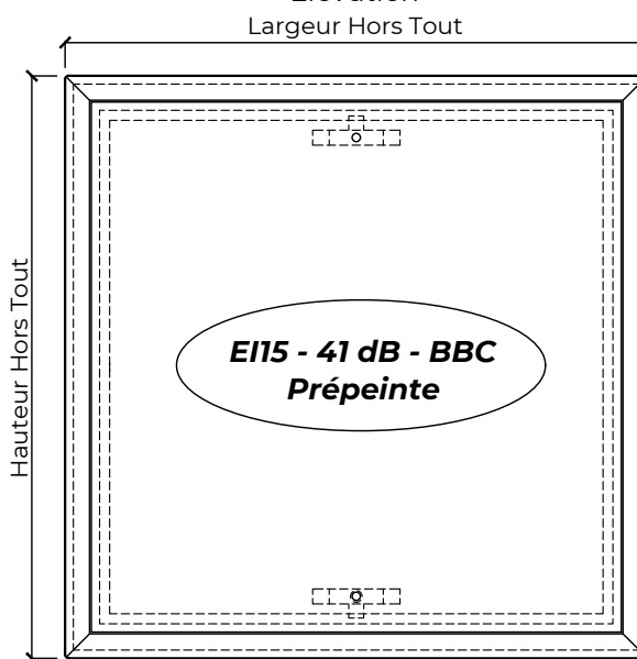
Élévation
