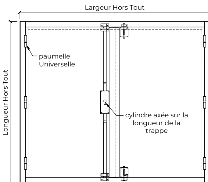
Elévation
