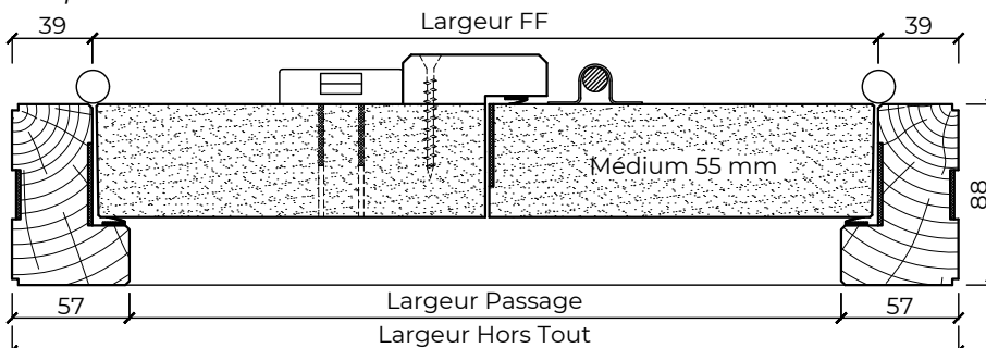
Coupe horizontale
