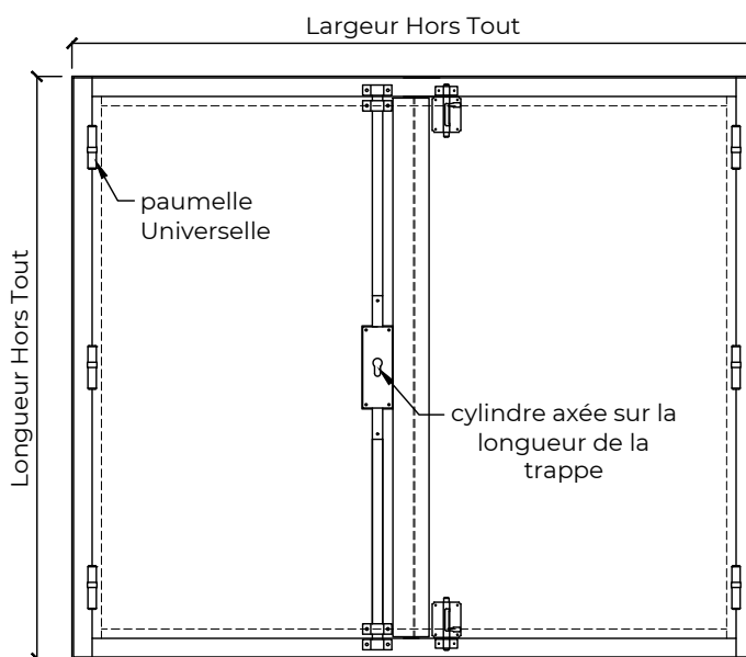
Elévation
