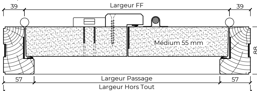
Coupe horizontale
