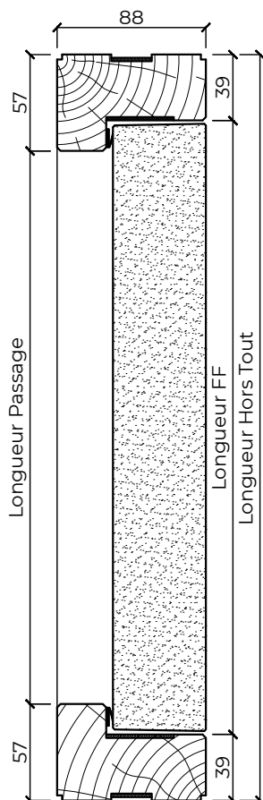
Coupe verticale
