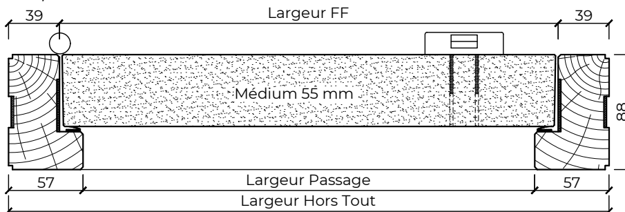
Coupe horizontale
