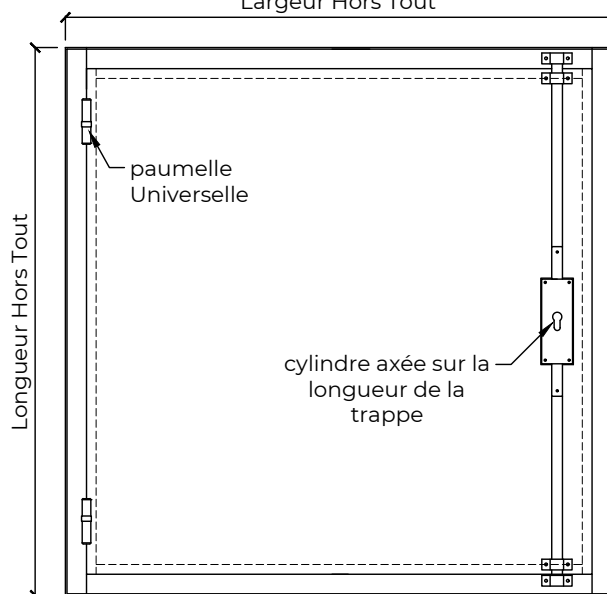
Elévation
