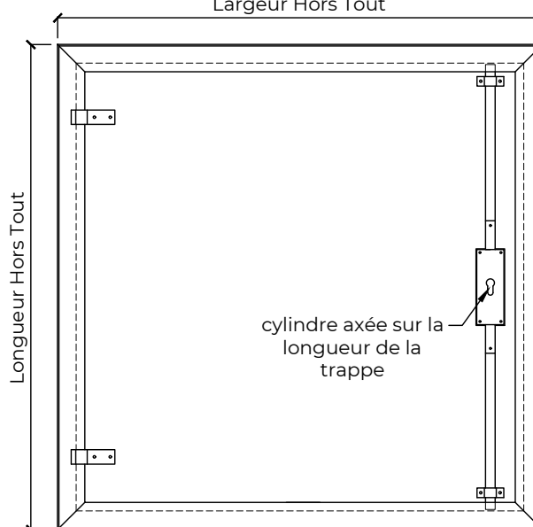
Elévation
