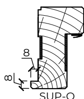
Option feuillure
