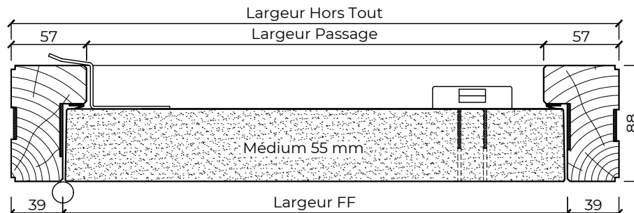
Coupe horizontale
