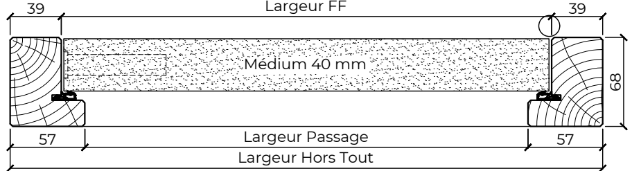
Coupe horizontale
