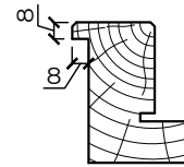
Option feuillure
