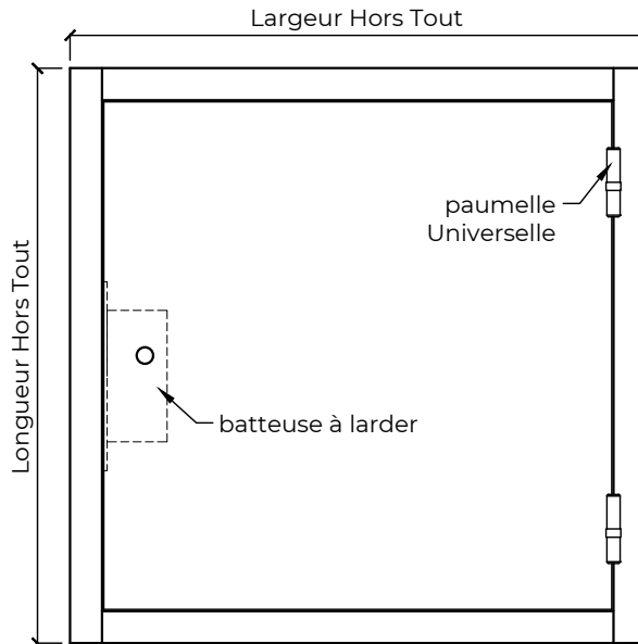
Elévation
