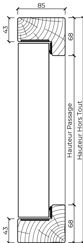
Coupe verticale
