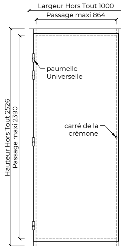
Elévation
