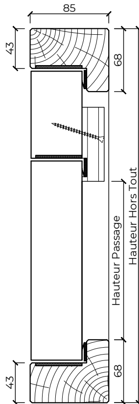
Coupe verticale
