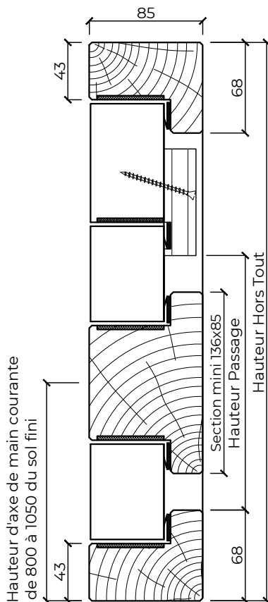
Coupe verticale
