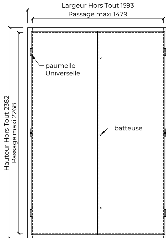
Elévation
