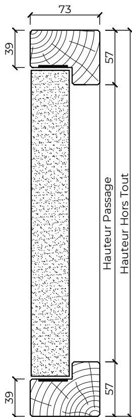
Coupe verticale
