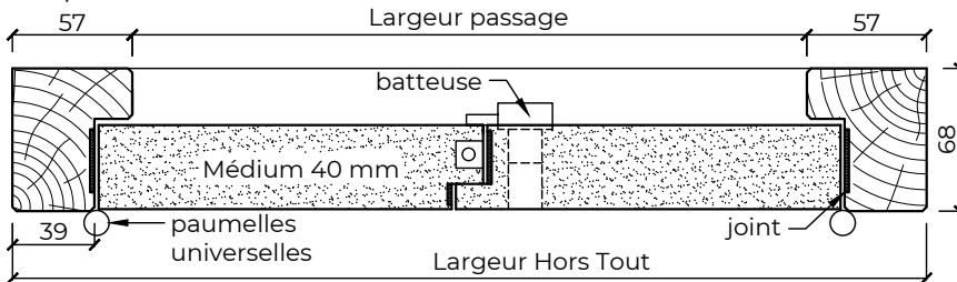
Coupe horizontale
