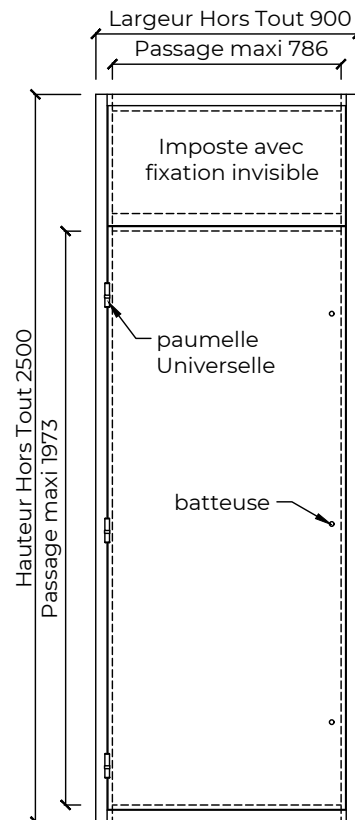
Elévation
