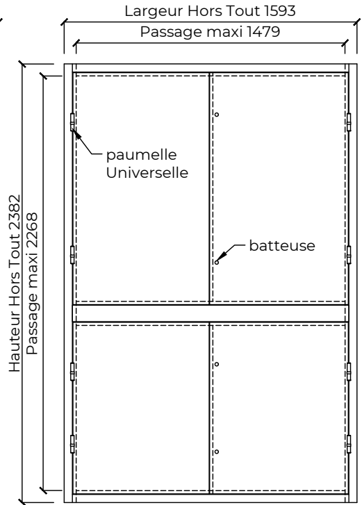
2 vantaux
