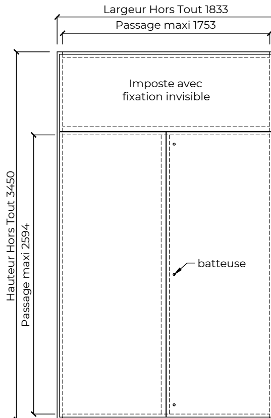
Élévation
