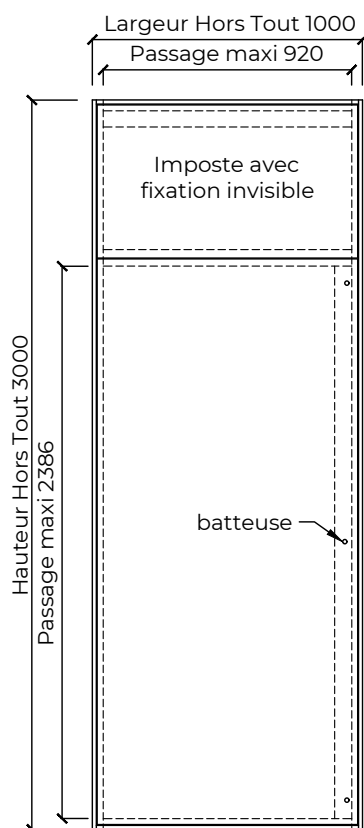
Élévation
