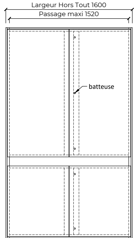
Elévation
