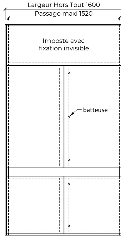
Elévation
