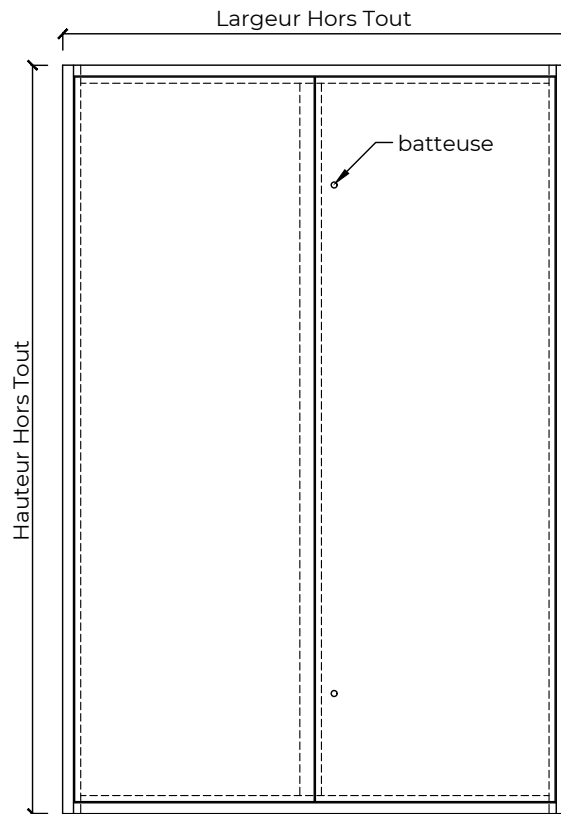
Élévation
