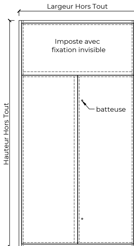
Élévation
