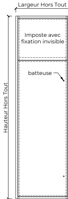
Elévation
