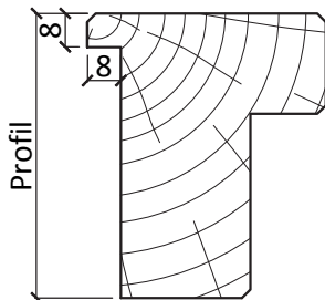
Suppression de joue côté feuillure
