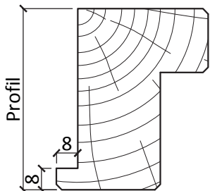
Suppression de joue côté opposé à la feuillure
