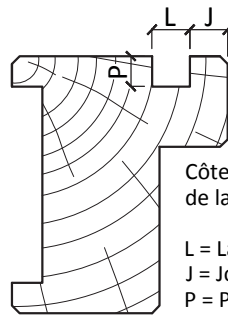
Rainure pour habillage d'embrasure
